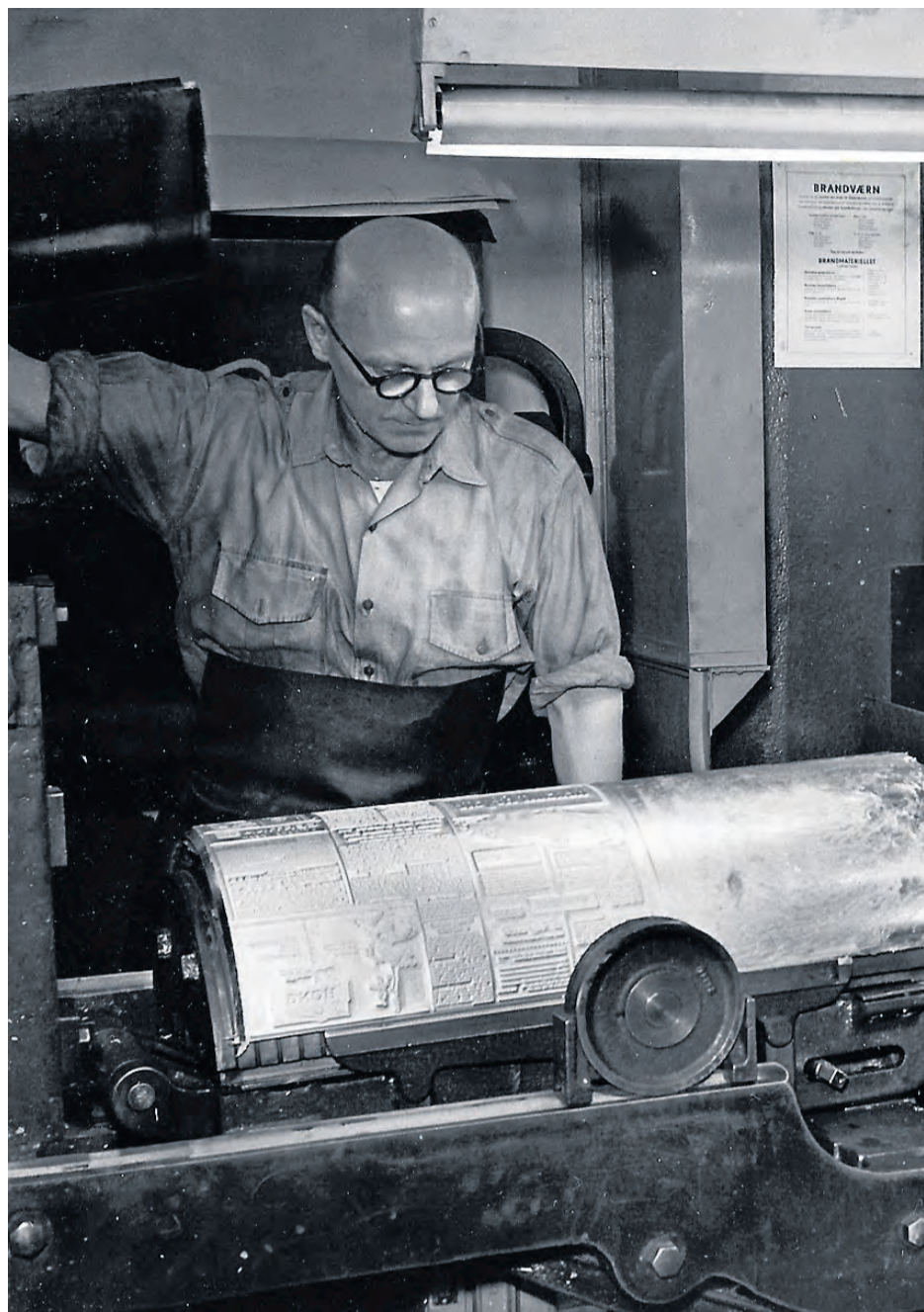
Støberiet på Nytorv, 1955. Færdigstøbt stereotypiplade kommer ud af Pony Autoplate-apparatet.
