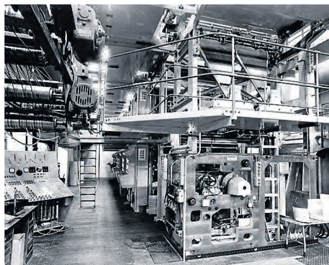
Den franske Marioni-maskine, som blev brugt til at trykke søndagstillægget - i farver. Foto: Max René
