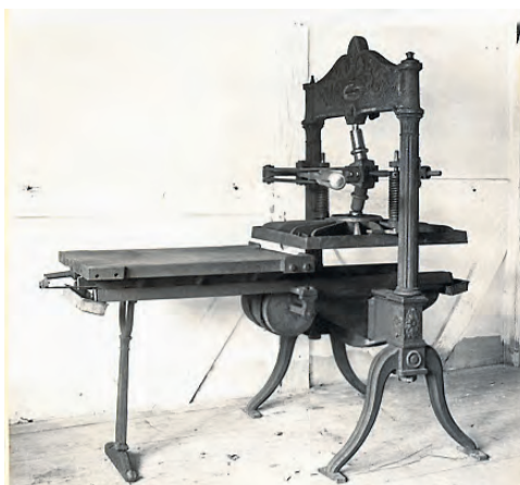
Hüttemeier-jernpressen. Billedet forestiller den originale presse, som findes opmagasineret i Aarhus. Foto: Den Gamle By
